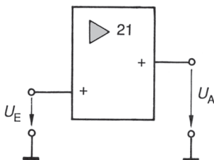
Obr. 6.19 Neinvertující zesilovač dle DIN 40 900 T 13
