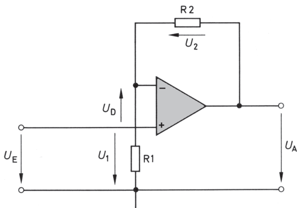
Obr. 6.18 Neinvertující zesilovač s OZ
