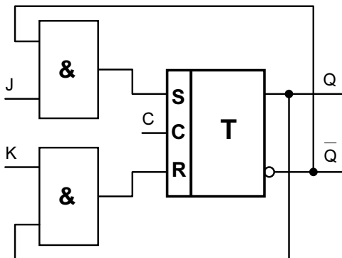
Obr. 4.19 Klopný obvod JK v blokovém tvaru
